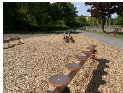
Fußsteller als federnde Balancierstrecke für die Körperbeherrschung
